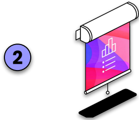
Import slides
